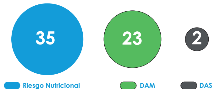
Figura 6. Niñas y niños detectados con un grado de desnutrición aguda o en riesgo nutricional durante junio
